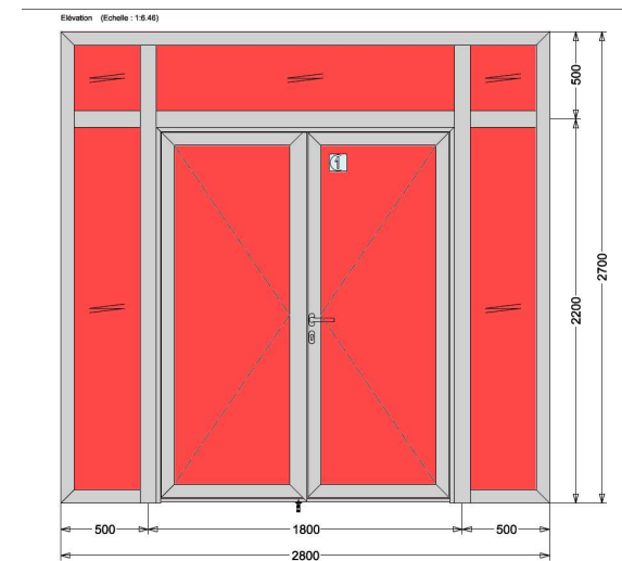
Châssis coupe feu Pare Flammes
