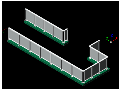
Modélisation et conception de Garde corps acier ou aluminium
