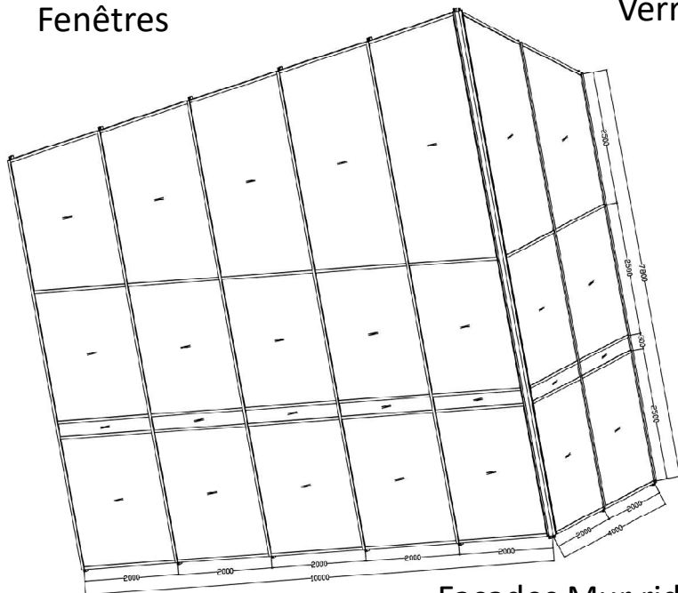
Façades Mur rideaux
