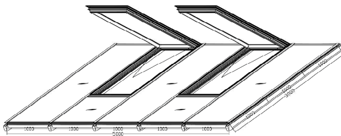
Verrières de Toiture
